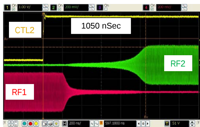
Figure 37. Switching Time [T AMB = -40°C, 3.3V]
