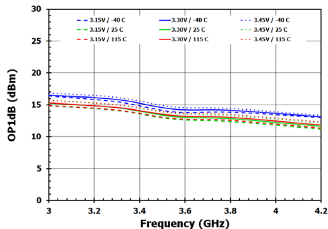
Figure 18. Output P1dB
