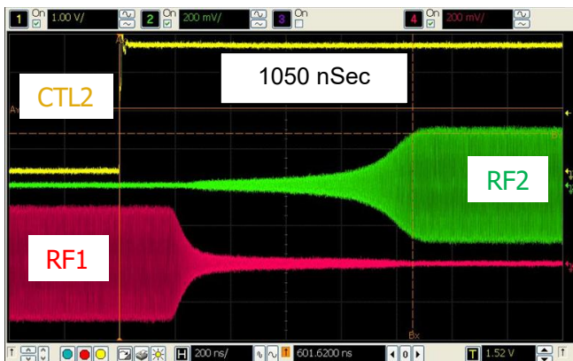
Figure 36. Switching Time [T AMB = 25°C, 3.3V]
