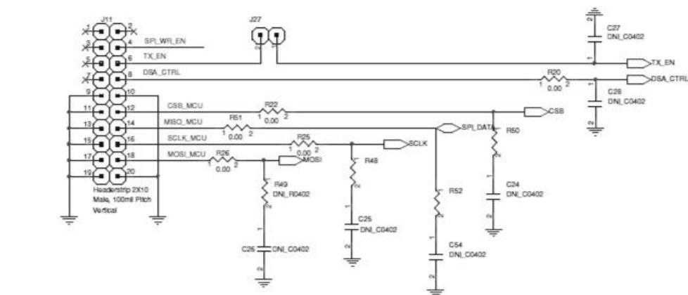
F2232H SPI MODULE (REVC) CONNECTOR 1 (2x10)
