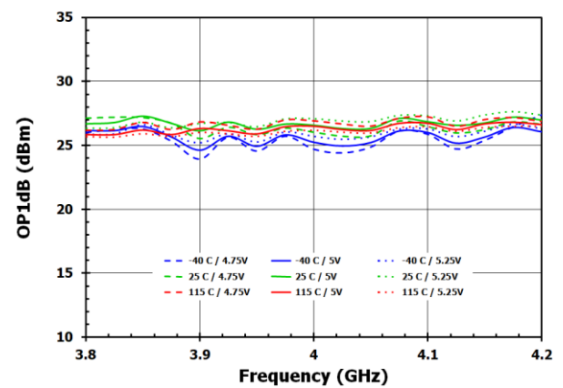
Figure 28. OP1dB
