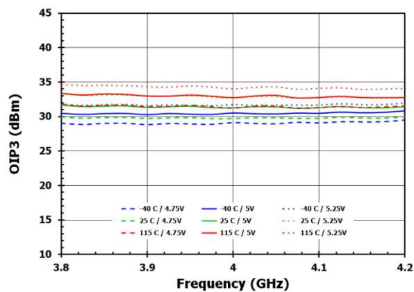
Figure 27. OIP3
