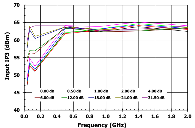
Input IP3
